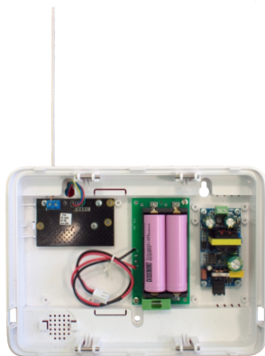
корпус с МБД, ИП и АКБ
